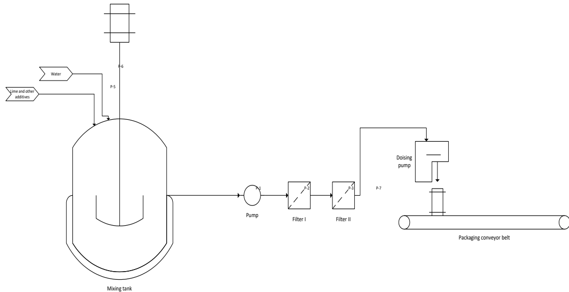
Figura 2. Proceso productivo
